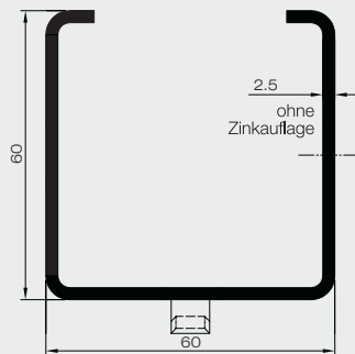
VA 60/60 END
