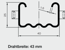
VA 40/25 SOLID
